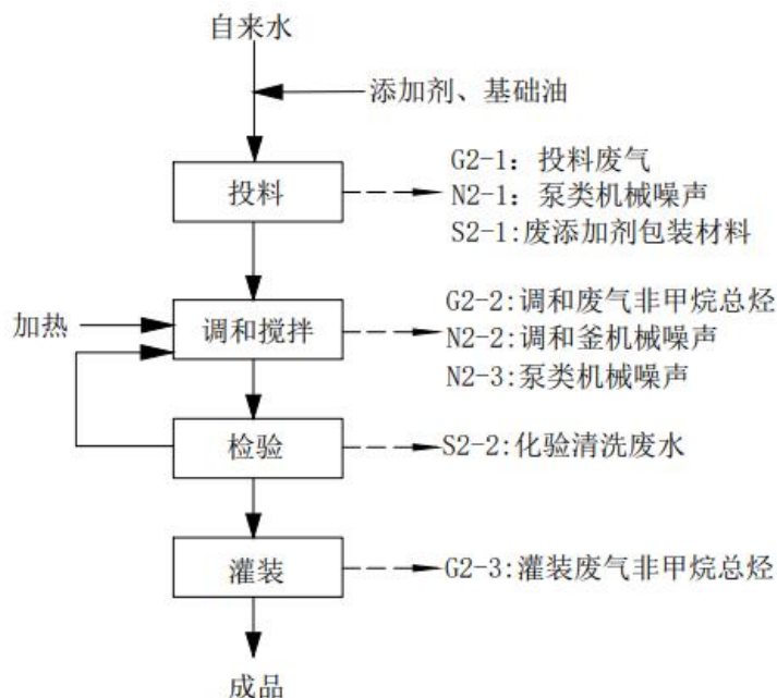
图2-3 水性金属加工油（液）工艺流程图
