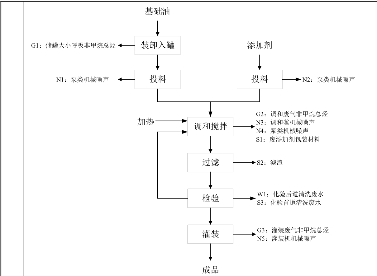
图2-2 润滑油调和工艺流程图
